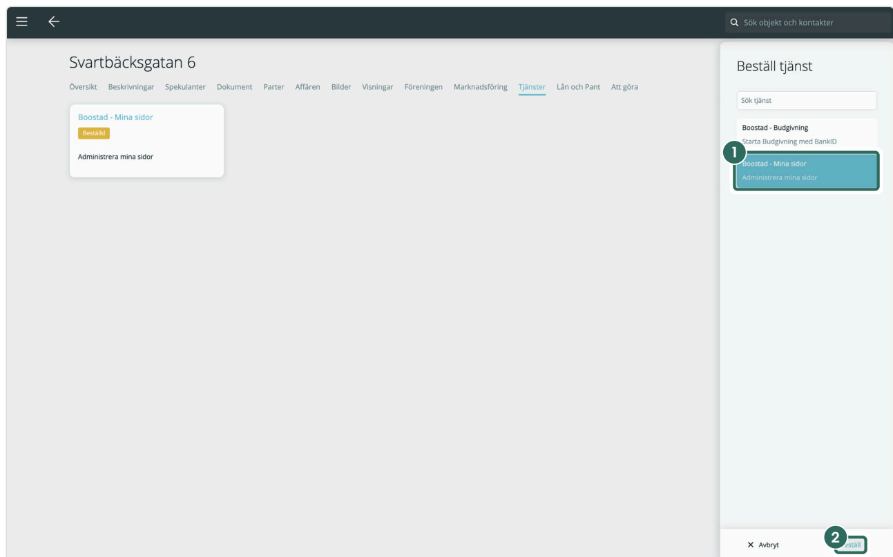
Bild 1. Fliken Tjänster på ett objekt i Vitec Express, med panelen Beställ tjänst.
